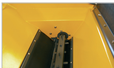
Das Epoke Dosiersystem: Umrührer, der evtl. Klumpen zerkleinert, und Auslegewalze für Dosierung.
